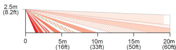
Figur 2: Sidovy
